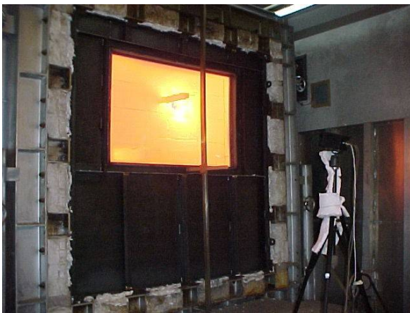
標準火災試験(Part 3)
